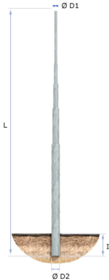
Palo rastremato h= 4m - Corpo illuminante viabilità pedonale
