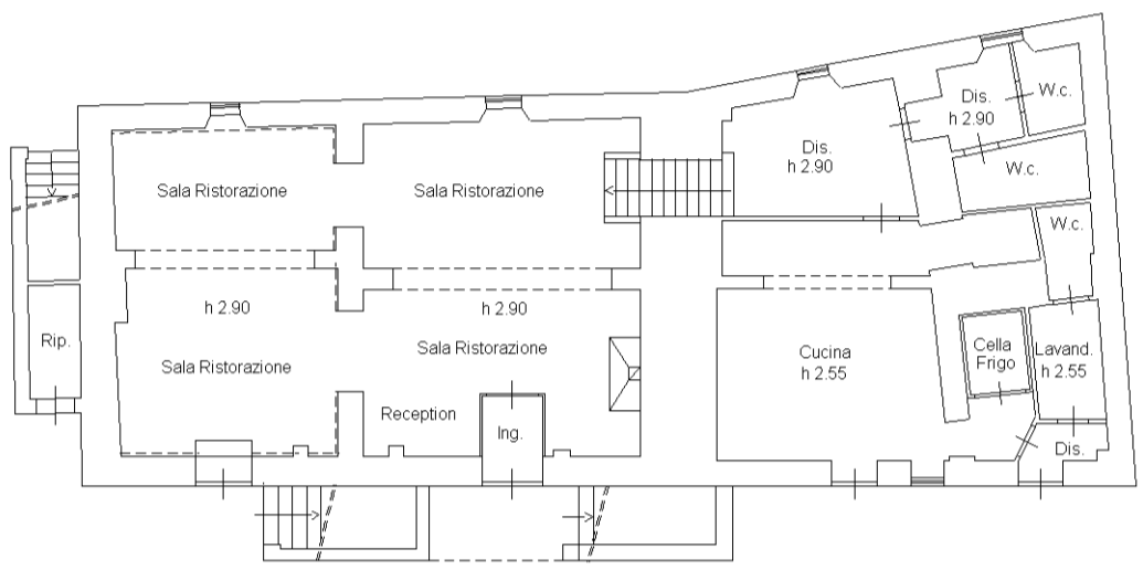
FABBRICATO "B" PIANO TERRA
