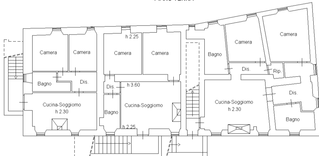
FABBRICATO "B" PIANO PRIMO
