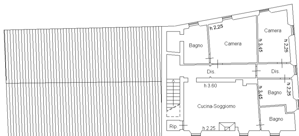
FABBRICATO "B" PIANO SECONDO
