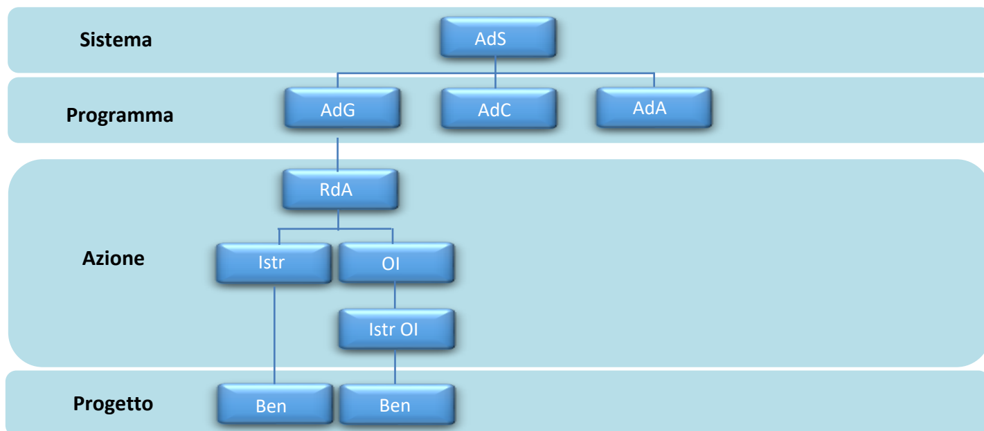
Figura 1 Gerarchia Utenti
